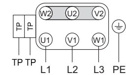
(Y) Schaltung / Star connection
